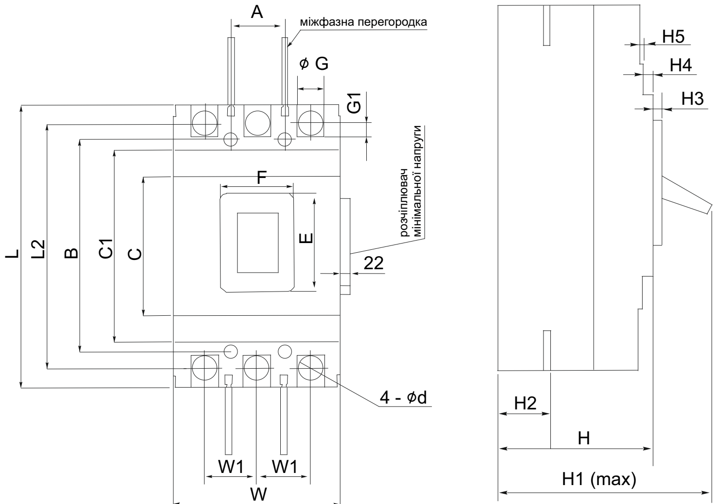
Рисунок 11 - Габаритні та настановні розміри вимикачів ВА44-400
