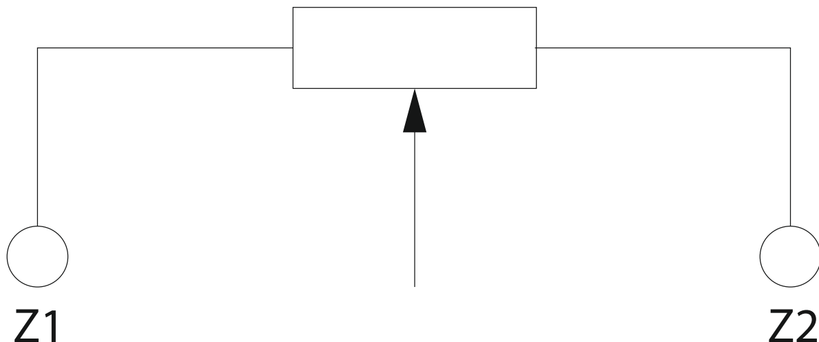
Рисунок 1 - Електрична схема підключення потенціометра
