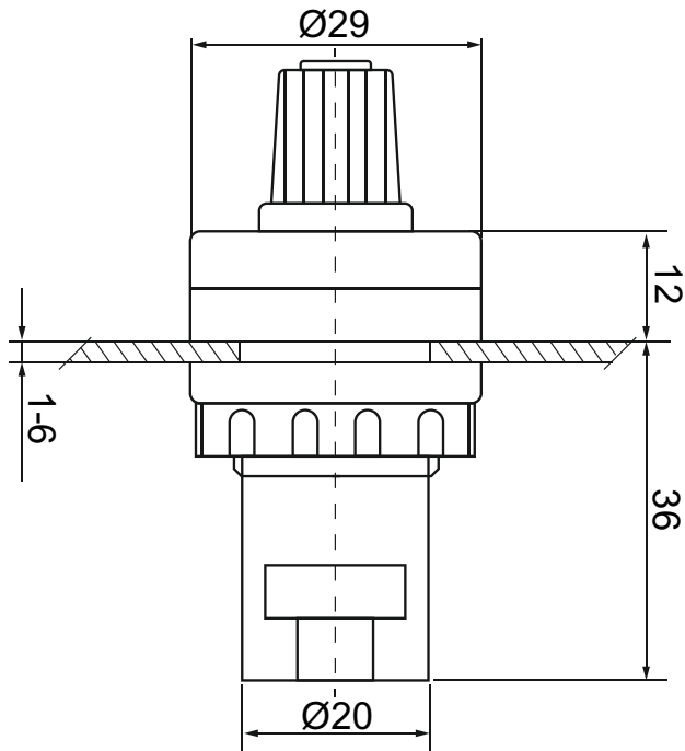
Рисунок 2 - Габаритні та настановні розміри потенціометра
