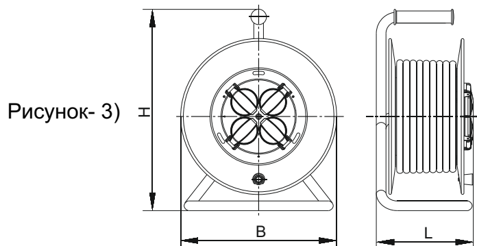
Котушка УК50к, УК50км
