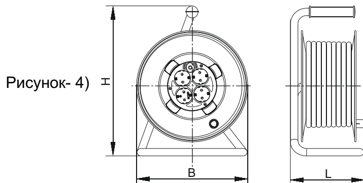
Котушка УК50+1
