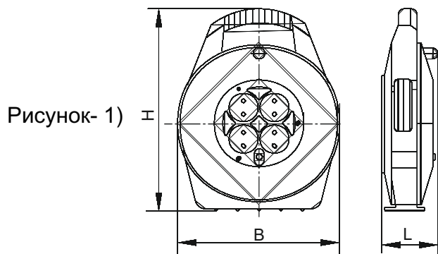
Котушка УК10
