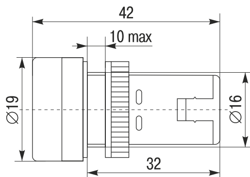
Рисунок 2 - AD16DS (LED)
