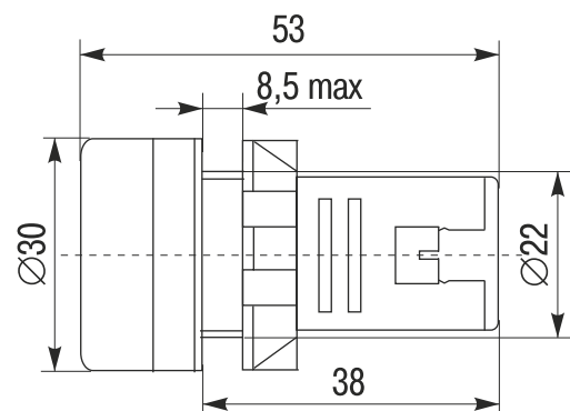
Рисунок 3 - AD22DS (LED)
