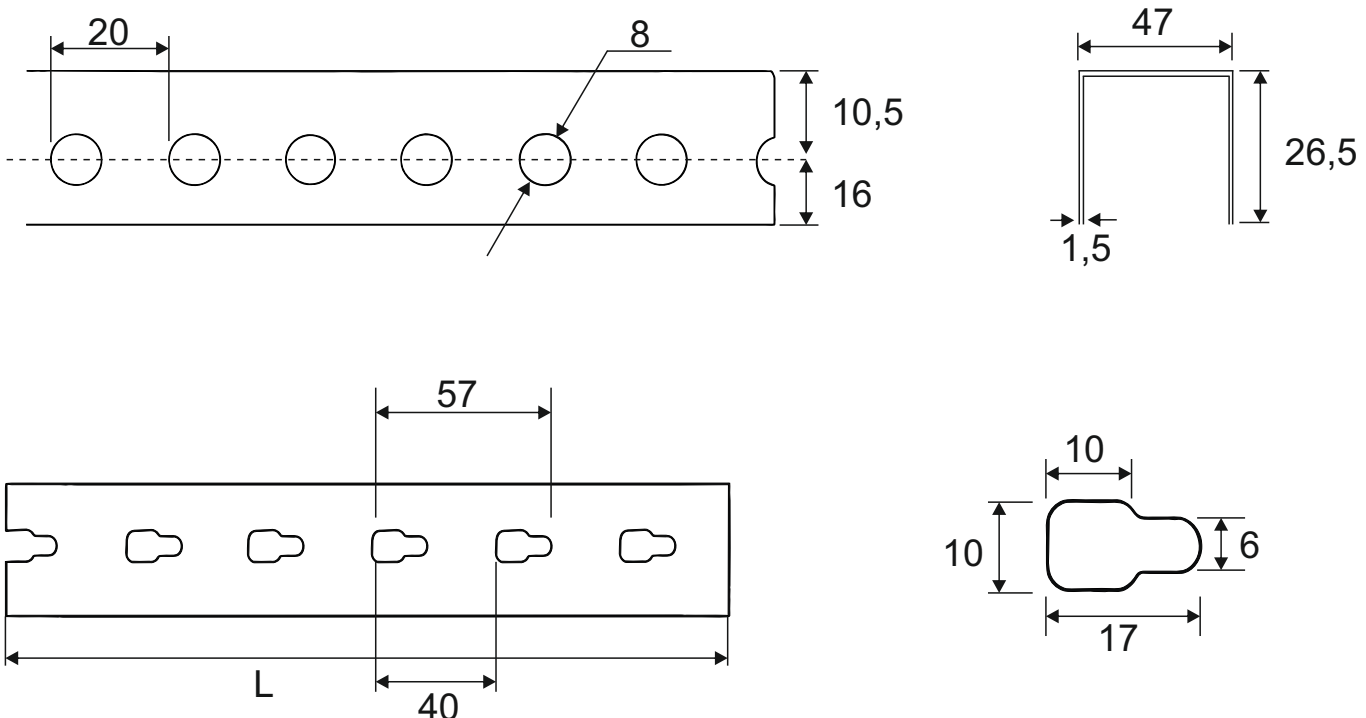
Малюнок 1 - Профіль перфорований П-подібний
