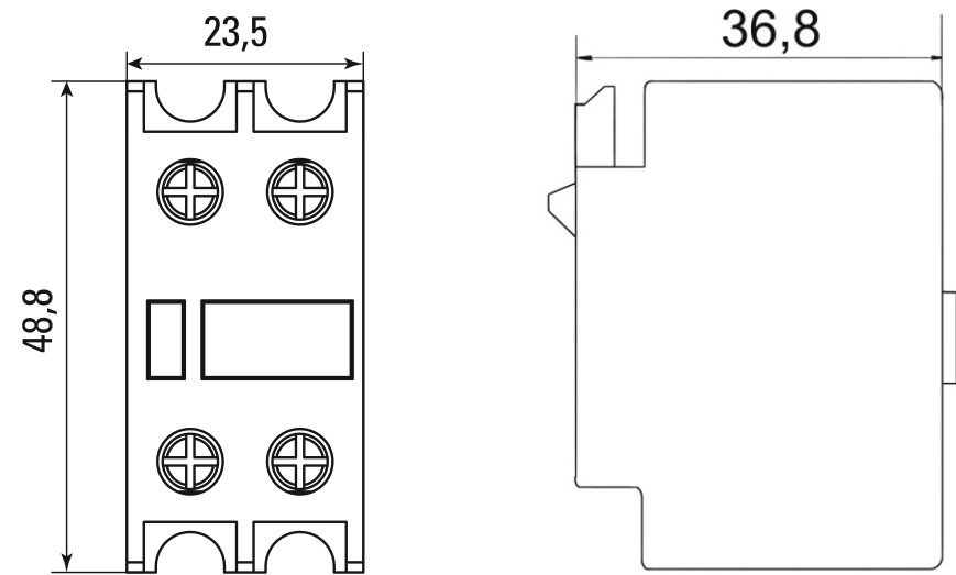
Мал. 1 Габаритні розміри ПК-11, ПК-20, ПК-02
