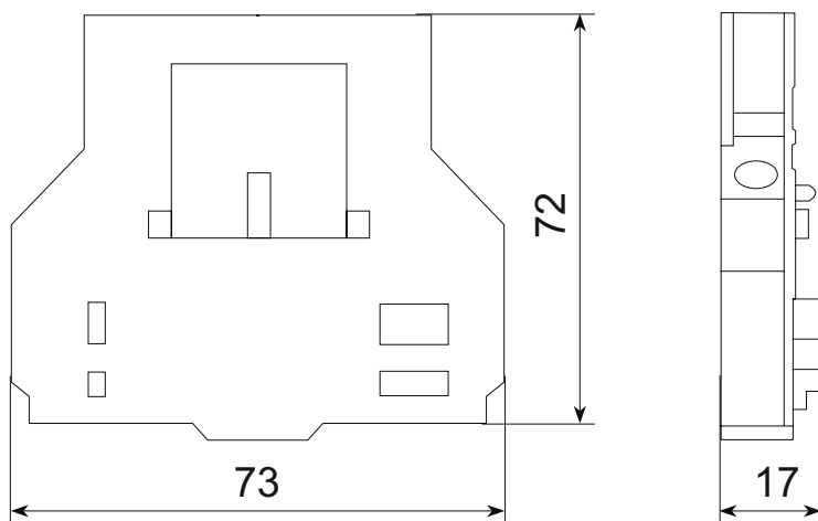
Мал. 3 Габаритні розміри ПКБ-02, ПКБ-11, ПКБ-20
