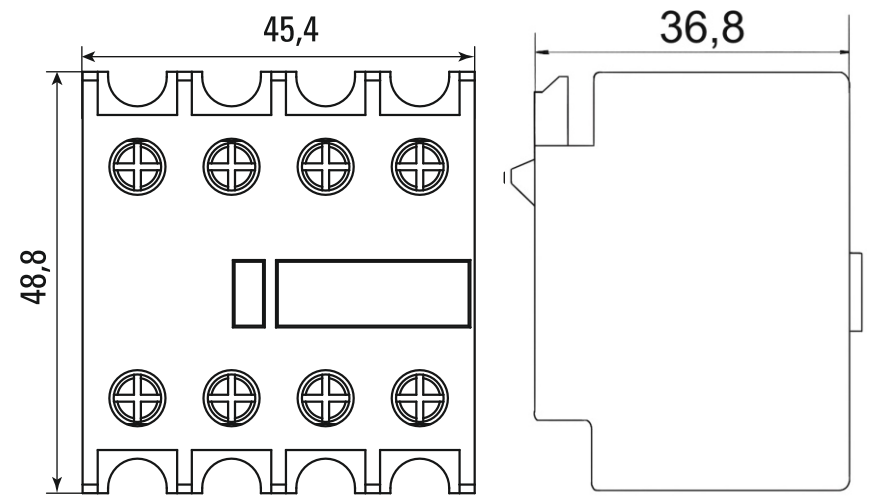
Мал.2 Габаритні розміри ПК-22, ПК-40, ПК-04
